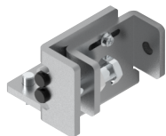
吊滑輪固定擋片 4 個 STOPER -4PCS (IN PROFILE)
