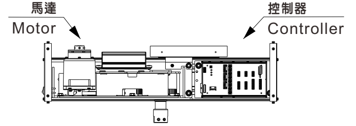
內拉式按裝示意圖 Operator
