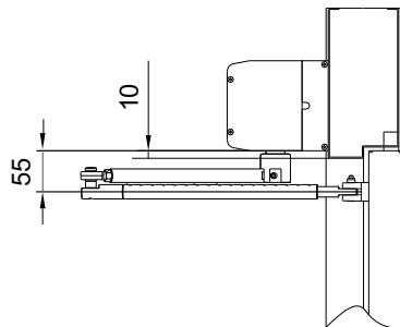
外推式開門方向(右側開門) Mounting
