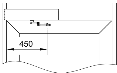
外推式推桿按裝尺寸圖
