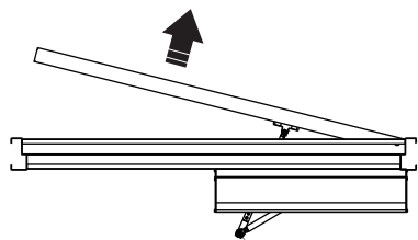
外推式開門方向(右側開門) Mounting
