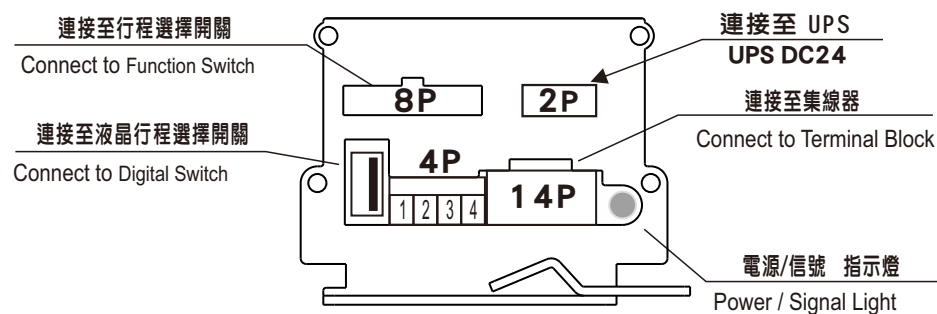
4P 插頭 4P terminal
